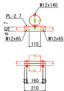
ビームパイプ接続部詳細図
