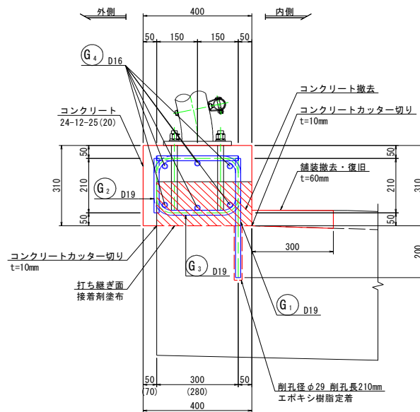
断面図 (3-3)
