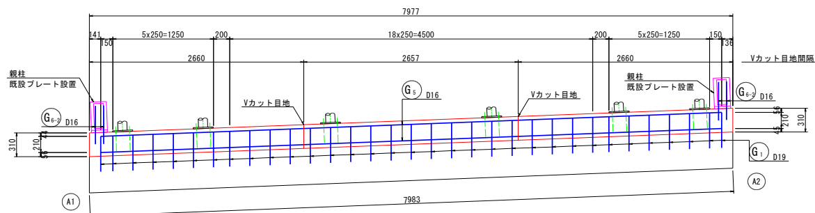
下流側側面図 (2-2)
