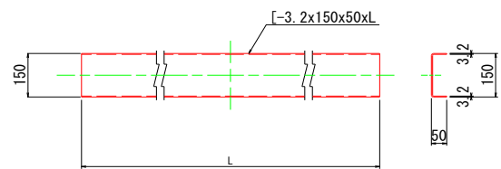
笠木詳細図
