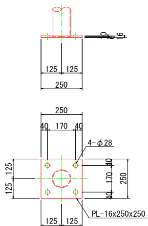
ベースプレート詳細図
