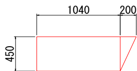
下流側型枠設置図
