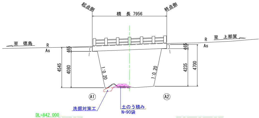
洗堀対策工施工時 側面図
