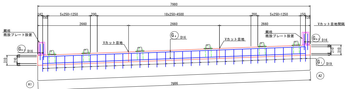
上流側側面図 (1-1)
