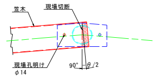
笠木加工詳細図
