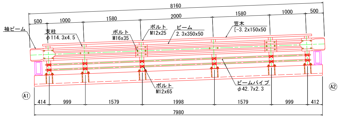
上流側側面図 (1-1)
