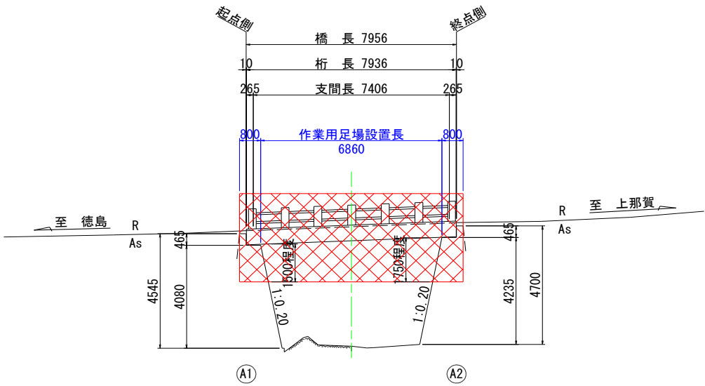
側面図
