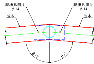
支柱部笠木詳細図
