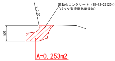
下流側型枠設置図
