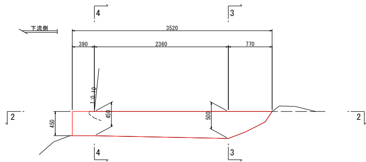
A1橋台基部展開図(1-1)
