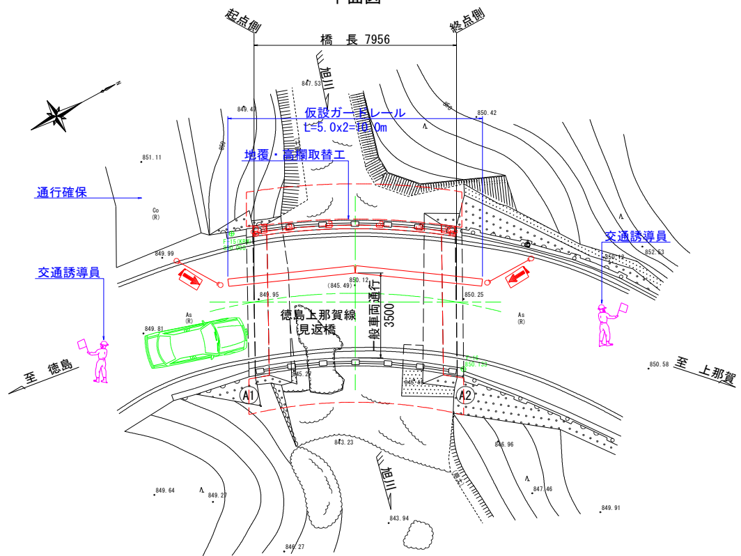
平面图
