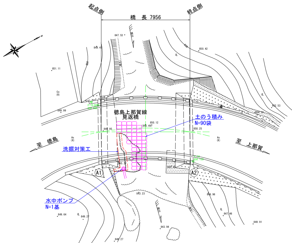
平面图
